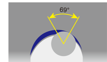
接觸啮合角度由 46^\circ 增加至 69^\circ
