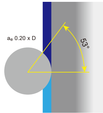
側銑切削啮合角度固定 53^\circ
