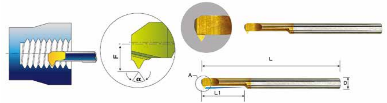
MIR 微型車刀 (60° 螺紋加工)
