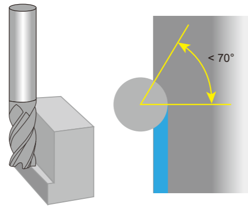
Tool angle of engagement & tool contact time 刀具切削啣合角度 & 刀具接觸時間
