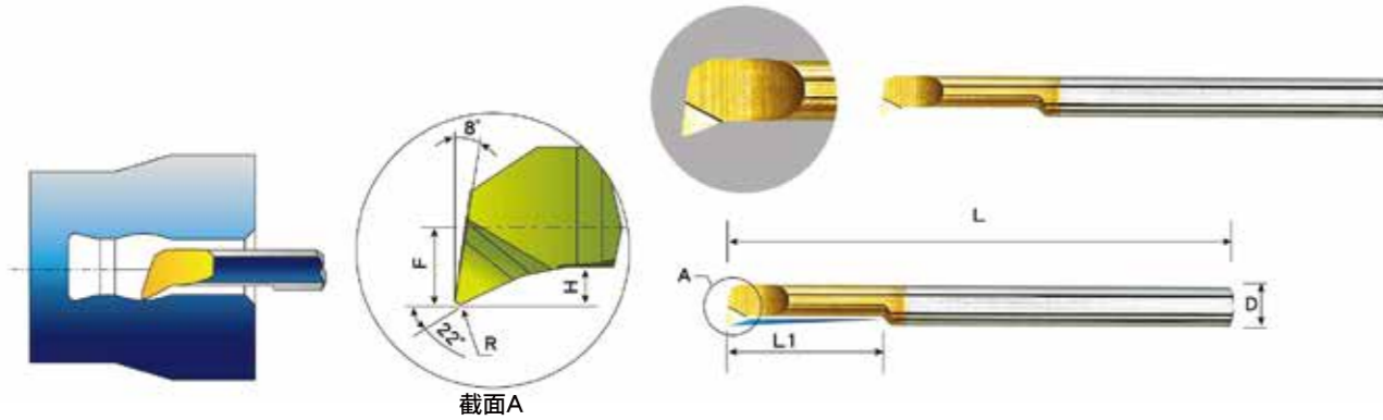
MPR 微型車刀 Micro Turning Cutter
