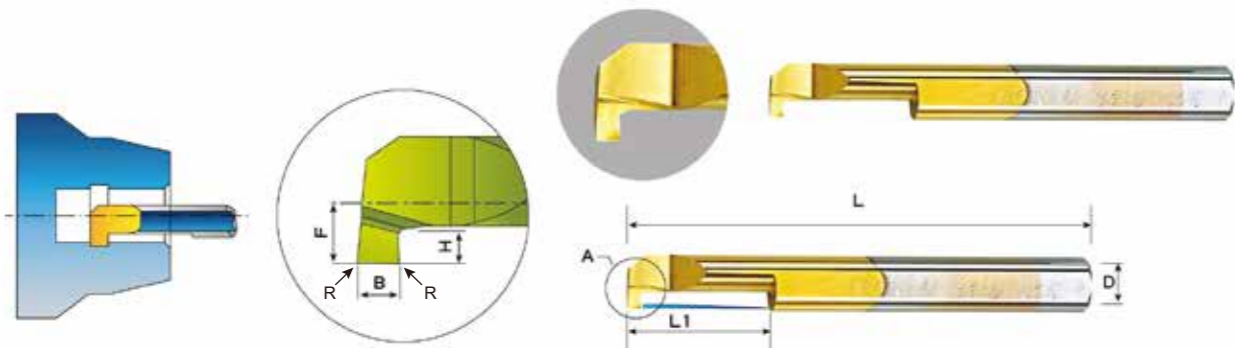
MGR 微型車刀(切槽) Micro Turning Cutter (Recessed)
